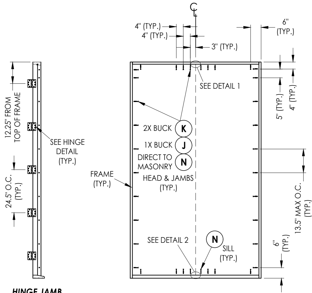
HINGE JAMB
